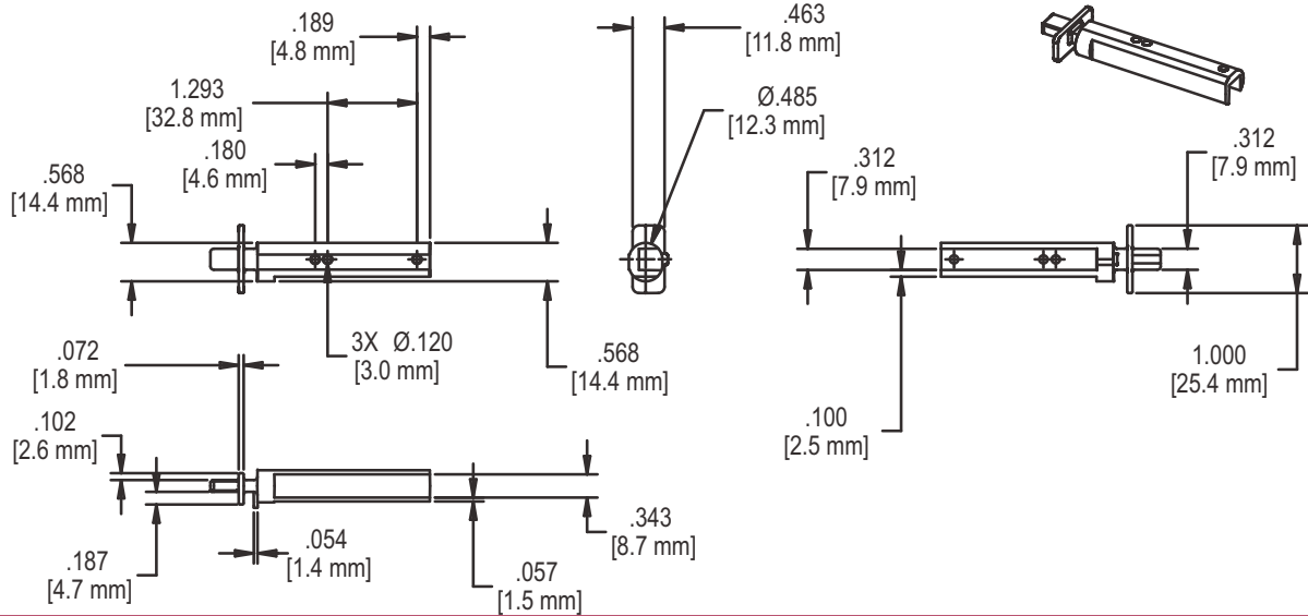
FIG. 6 32794 PIVOT BAR
